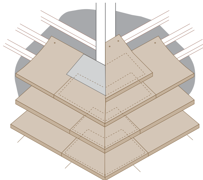
Mitred hip
